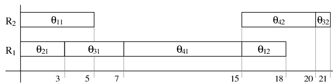
(c) Construcción de la planificación mediante SSGS. Paso 2
