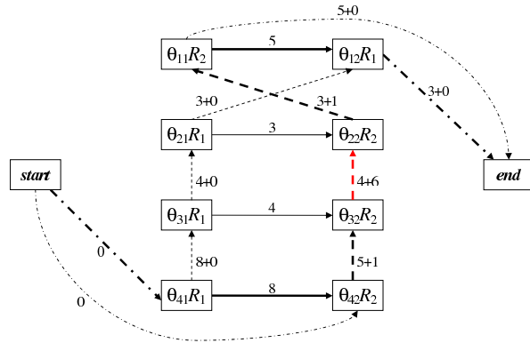
(a) Grafo disyuntivo de la planificación original
