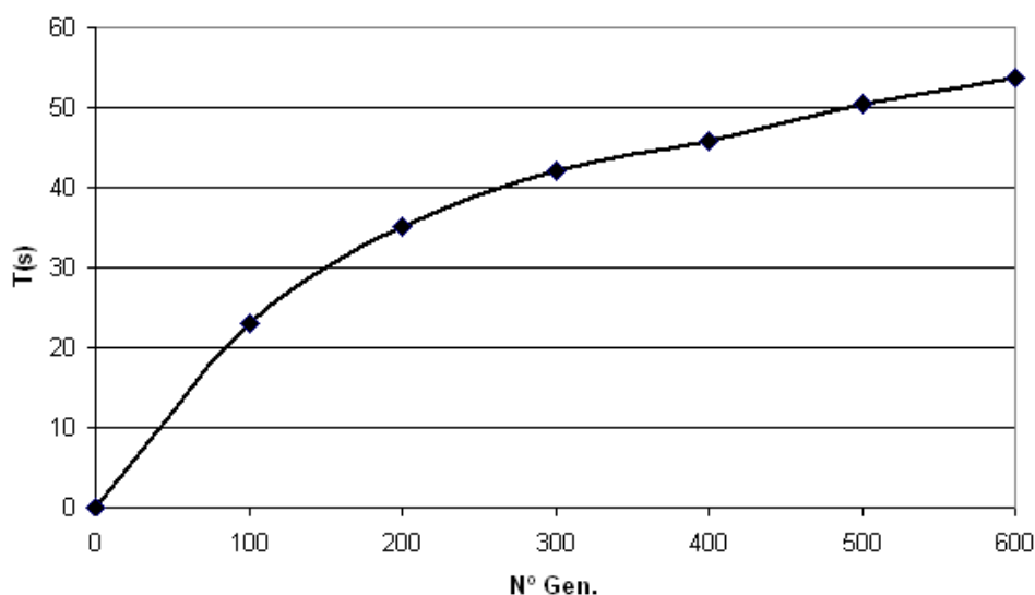
Figura 8.1: Experimentos makespan: Convergencia del algoritmo genético híbrido. Evolución del tiempo según el número de generación
