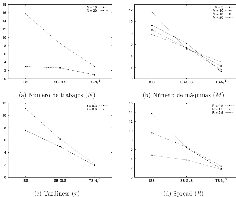
Figura 9.1: Experimentos maximum lateness: Interacción entre parámetros y algoritmos, con el error respecto a la mejor solución conocida en el eje Y
