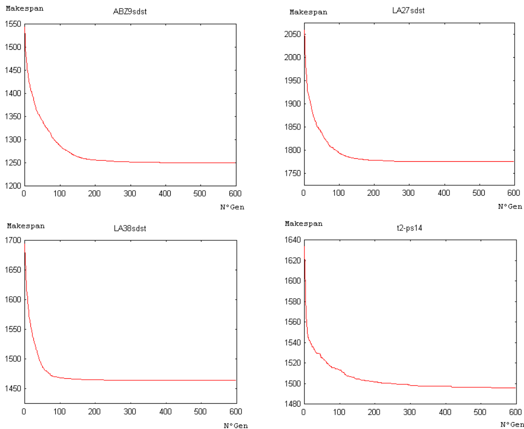
Figura 8.2: Experimentos makespan: Convergencia del algoritmo genético híbrido. Evolución del makespan según el número de generación
