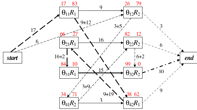
(a) Grafo disyuntivo de la planificación inicial
