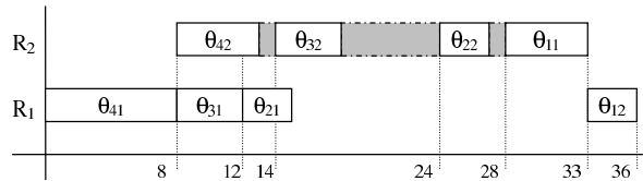
(b) Diagrama de Gantt de la planificación original
