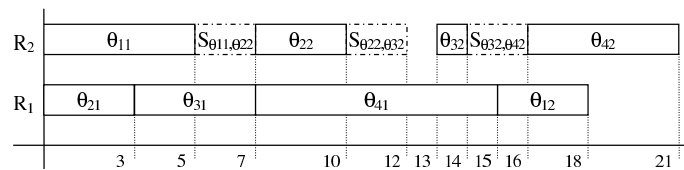
Figura 3.3: Contraejemplo 2: SSGS genera una planificación que ni siquiera es semiactiva
