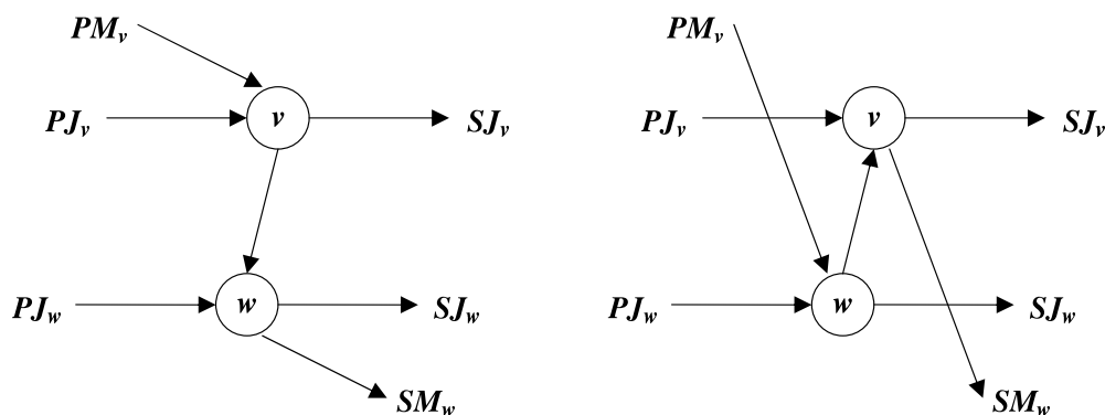
Figura 7.8: Inversión de un arco en un bloque crítico
