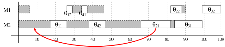
(b) Diagrama de Gantt de la planificación inicial
