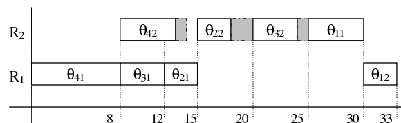
(d) Diagrama de Gantt de la planificación vecina
