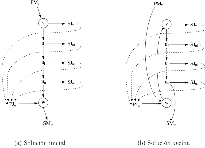
Figura 7.4: Posibles caminos alternativos que pueden existir en un bloque crítico, que darían lugar a un ciclo tras mover la operación w antes de la operación v
