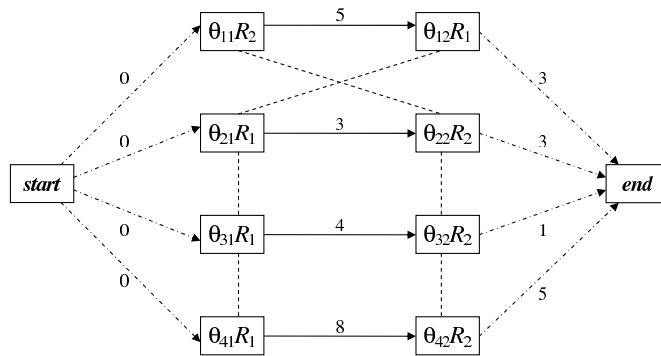
(a) Grafo disyuntivo de la instancia
