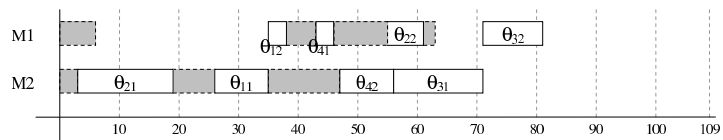
(d) Diagrama de Gantt de la planificación vecina
