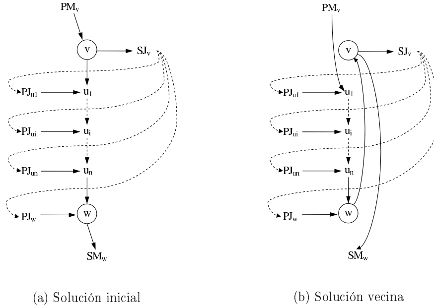
Figura 7.5: Posibles caminos alternativos que pueden existir en un bloque crítico, que darían lugar a un ciclo tras mover la operación v después de la operación w
