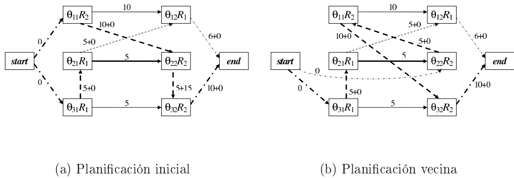
Figura 7.6: Utilización de todos los caminos críticos con la estructura N_1^S
