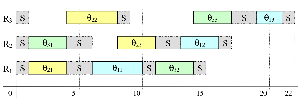
Figura 2.4: Diagrama de Gantt para la planificación representada en la figura 2.1
