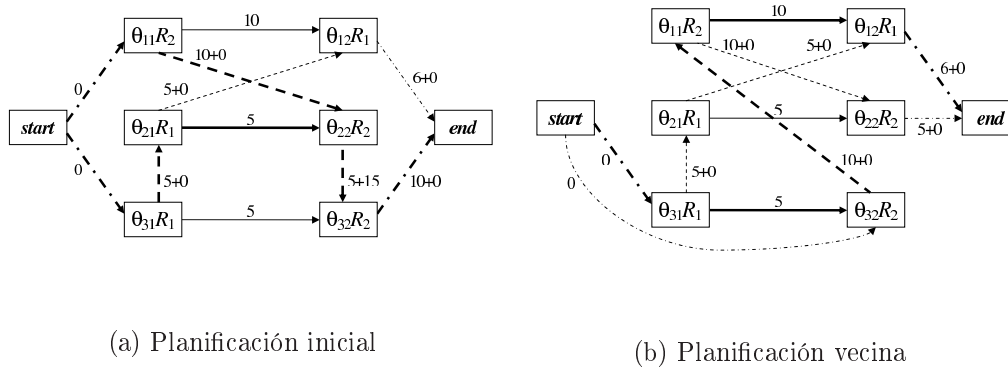
Figura 7.7: Utilización de todos los caminos críticos con la estructura N^S
