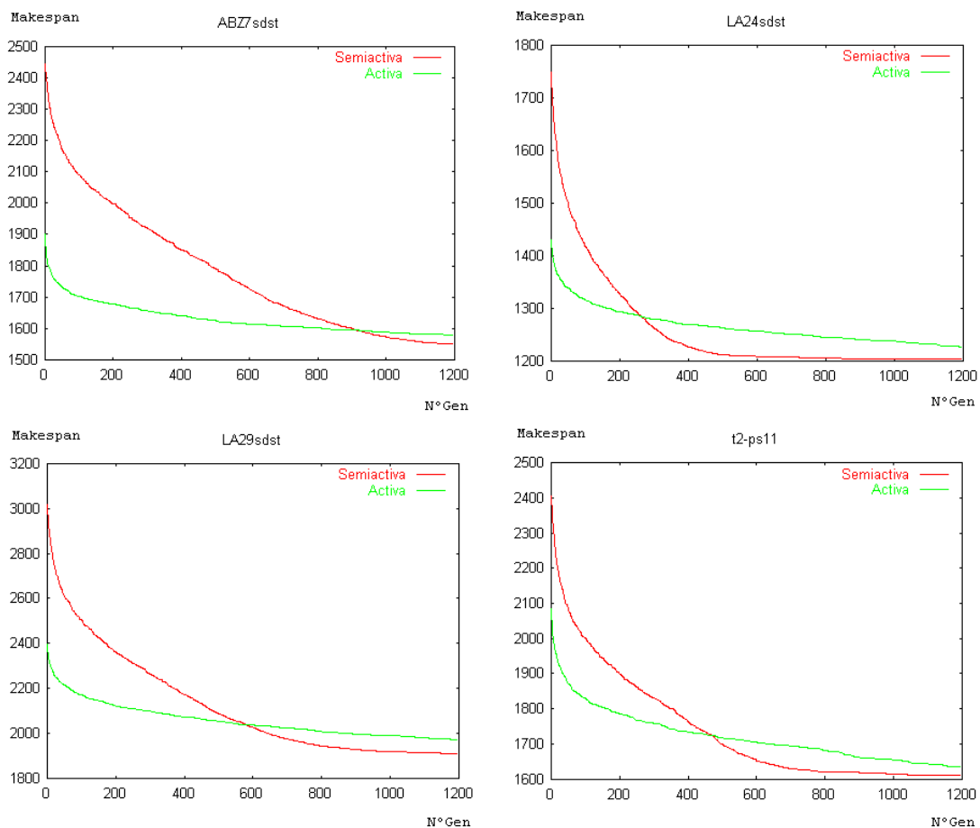
Figura 8.3: Experimentos makespan: Planificaciones semiactivas frente a activas en un algoritmo genético. Evolución del makespan según el número de generación
