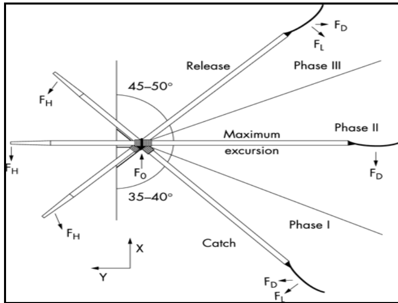
Fig. 3. Fuerzas que actúan sobre la pala durante la fase acuática, donde F_H es la fuerza aplicada por las manos del remero, F_D la resistencia que ejerce el agua sobre la pala, F_L la fuerza que tiende a levantar la pala del agua, F_0 las fuerzas de reacción en el anclaje del remo. Tomado de Badouin A y Hawkins D 25 .
