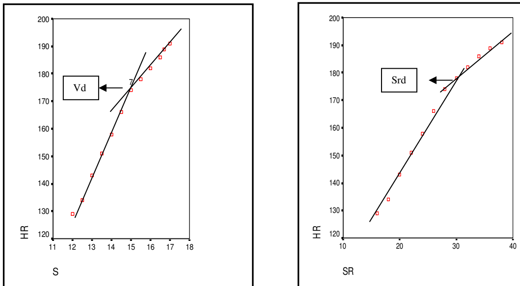
Gráfico 4. Cálculo mediante regresiones lineales del punto de deflexión de la velocidad (Vd) y de la frecuencia de paladas (Srd) durante un test de Conconi., donde HR es la frecuencia cardíaca, S es la velocidad de la embarcación y SR la frecuencia de paladas.
