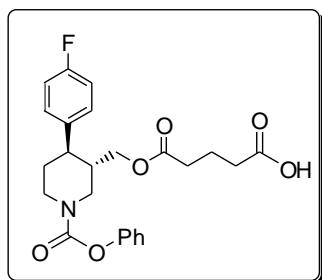
(3 S ,4 R )- 5b
