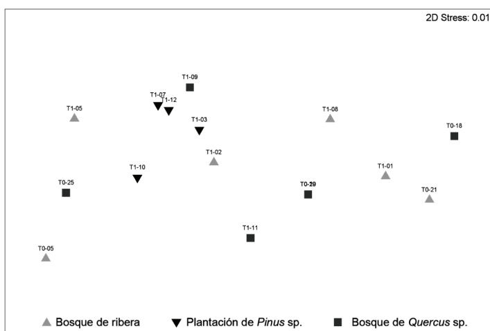
Fig. 2. Análisis de escalamiento multidimensional no métrico (MDS) de las comunidades de opiliones forestales edáficas de la cuenca media-alta del río Tâmega. / Non-metric multi-dimensional scaling (MDS) analysis of the ground-dwelling forest harvestmen communities from middle-upper basin of Tâmega River.
