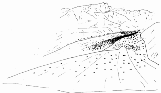
Fig. 2 Incisión sobre las gonfolitas que alberga dos niveles encajados de terraza. De ellos, el más elevado enlaza con un cono de deyección que alcanza el fondo de valle (este modelo se repite en la desembocadura de las principales canales).
