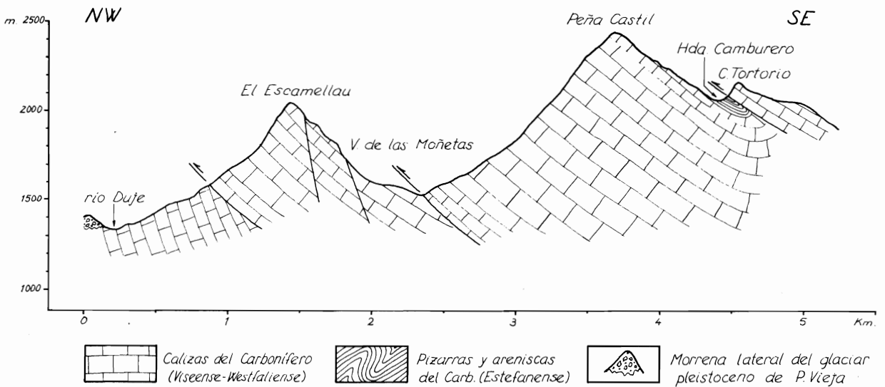
Fig. 1 Corte geológico desde el Escamellau hasta el Cabezo Tortorio. La misma disposición en escamas puede verse en la fotografía de la fig. 7.
