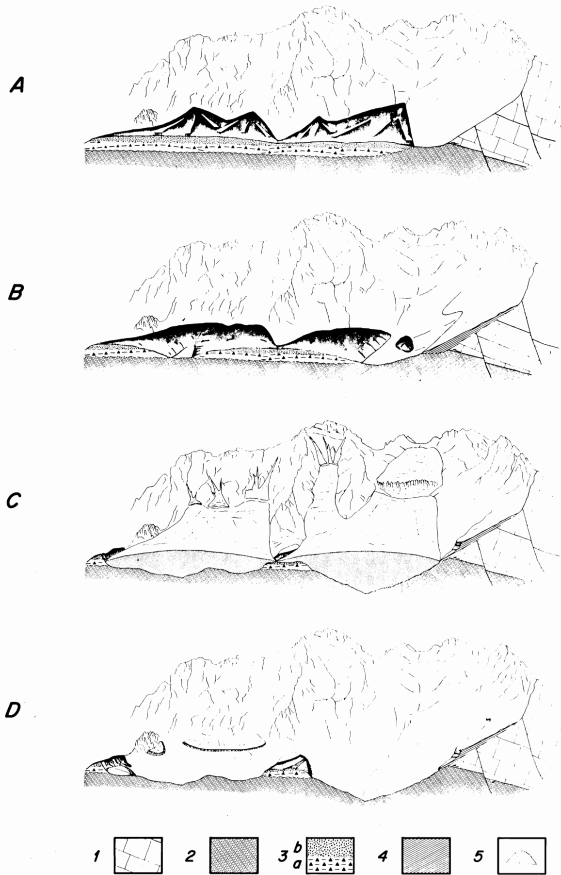
Fig. 3 Esquema evolutivo de la cabecera del Duje (Peña Vieja y Puertos de Aliva). LEYENDA: Litología: 1. Calizas de Montaña y de los Picos de Europa (NamurensesWestfalienses). 2. Pizarras, areniscas y calizas (WestfaliensesEstefanenses). Formaciones superficiales: 3. Derrubios homométricos estratificados (a) sobre derrubios heterométricos (b); ambos cementados. 4. Derrubios estratificados y cementados. 5. Morrenas de retroceso y de nevero. ETAPAS (de arriba a abajo): A) Primera fase de relleno de los terrenos deprimidos por grandes conos de derrubios en dos etapas menores. B) Excavación a partir de los ejes de las canales y segunda fase de aporte y cementación de derrubios. C) Excavación glacial. D) Elaboración de formas nivales al finalizar la etapa glacial.
