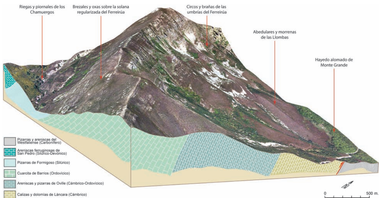
FIG. 10. El papel de la litología y la tectónica en las unidades de paisaje del pico Ferreirúa (Asturias-León): bloque-diagrama.
