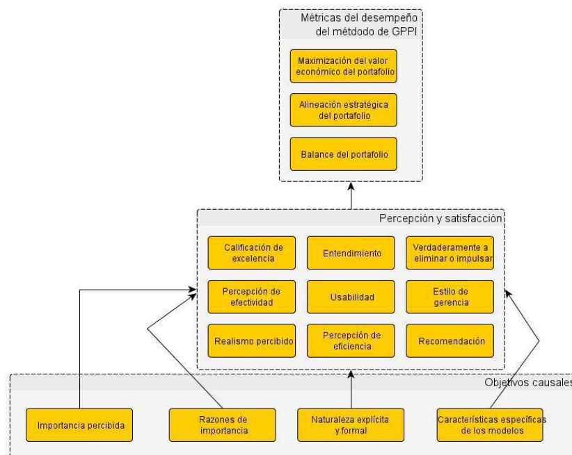
Figura 7.1 Desempeño de los métodos de GPPI
