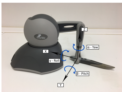
Figura 9: Representación de la orientación del lápiz del dispositivo háptico.
