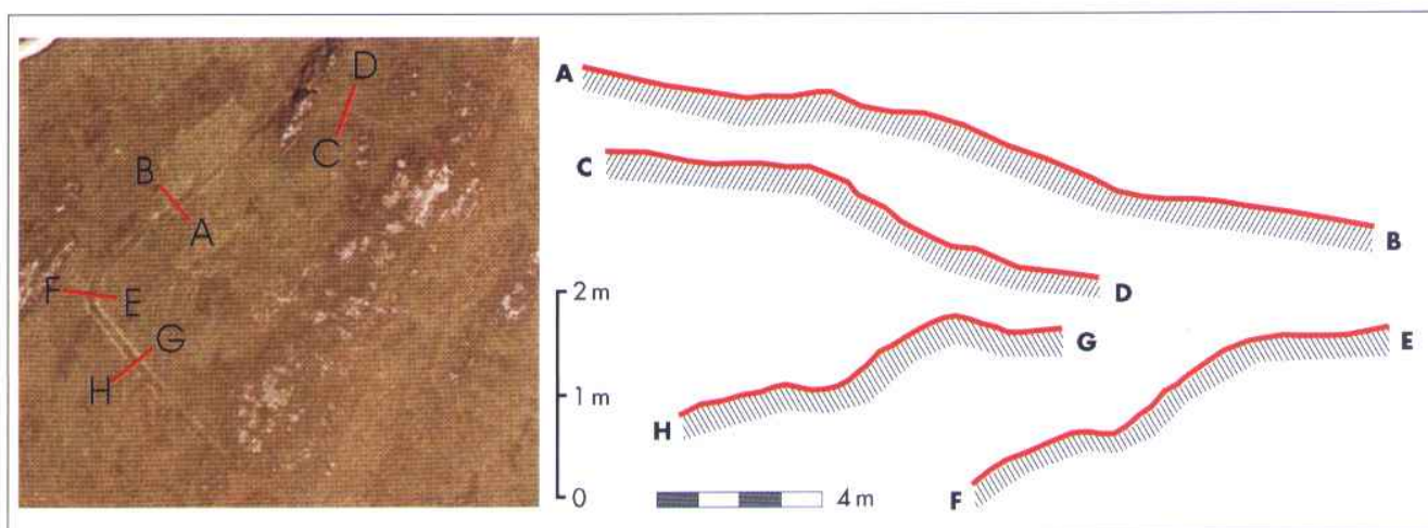
Secciones transversales a las estructuras de defensa en diferentes tramos de los límites del recinto.
