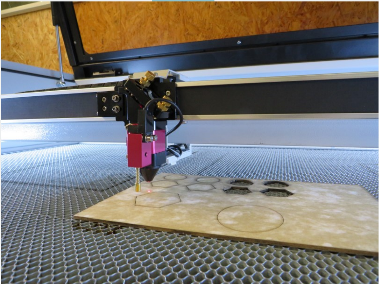
Cortadora láser
