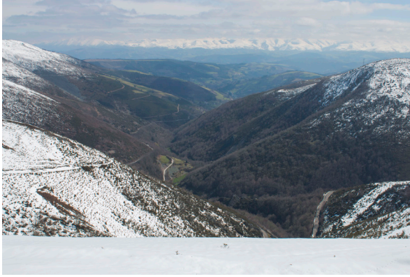
Fig. 3. Vista xeral do val de La Reigada dende o seu extremo occidental
